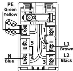
220-240V/380-415V 2L/1N~
