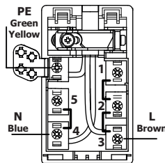
220-240V 1L/1N~
