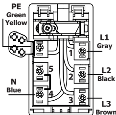
220-240V/380-415V 3L/1N~
