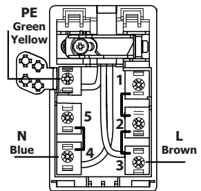
220-240V 1L/1N~
