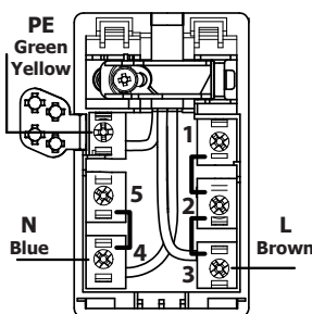
220-240V 1L/1N~
