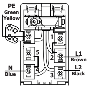
220-240V/380-415V 2L/1N~
