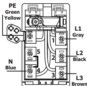
220-240V/380-415V 3L/1N~
