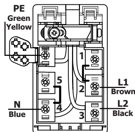
220-240V/380-415V 2L/1N~
