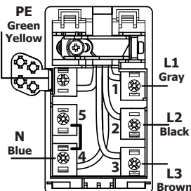
220-240V/380-415V 3L/1N~
