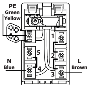
220-240V 1L/1N~
