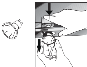
Fig. 27: Byte av GU10-lampa
